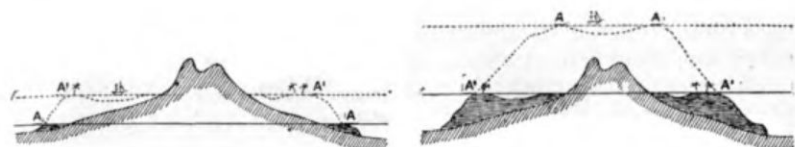
КОРАЛЛОВЫЕ ОБРАЗОВАНИЯ. АА — ОКАЙМЛЯЮЩИЙ РИФ, А'А' — БАРЬЕРН РИФ, А'А' — БАРЬЕРНЫЙ РИФ, —————> А'А'' — АТОЛЛ
